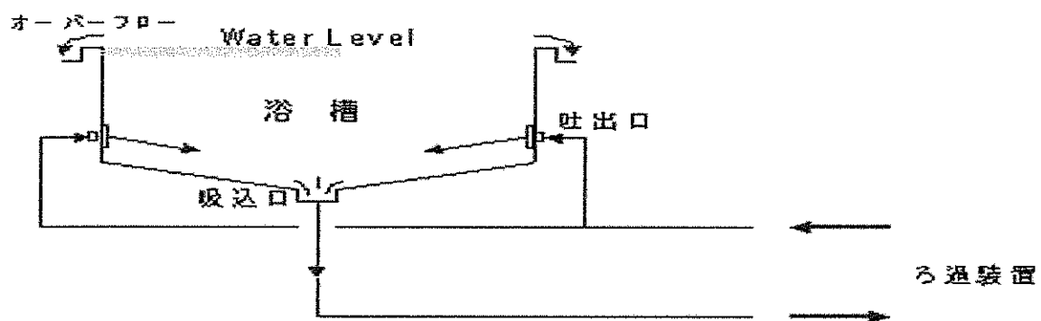
図-2 側壁吐出・底面還水方式
